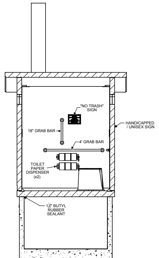
SECTION 2-2 SCALE 1 : 48
