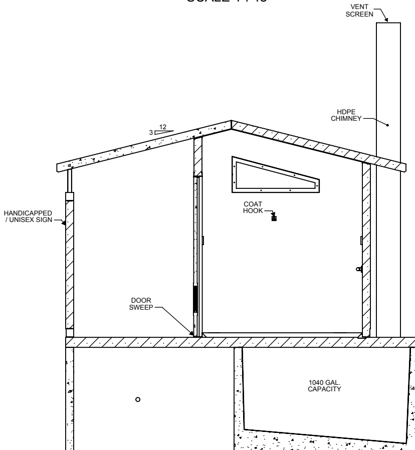
SECTION 1-1 SCALE 1 : 48
