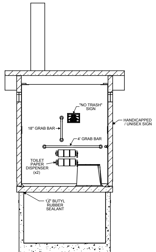
SECTION 2-2 SCALE 1 : 48
