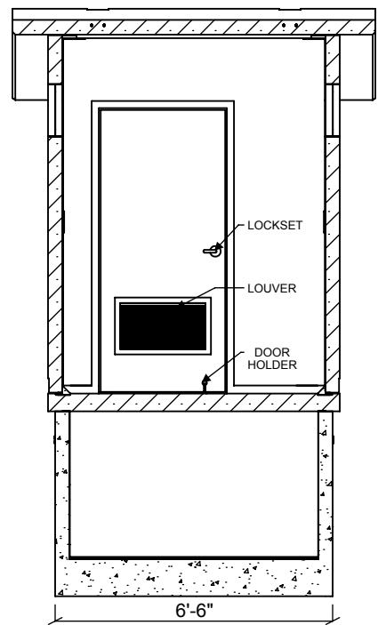
SECTION 2-2 SCALE 1 : 48
