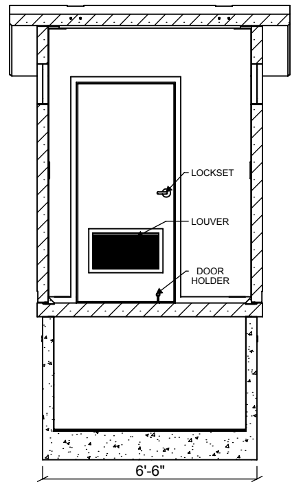
SECTION 2-2 SCALE 1 : 48
