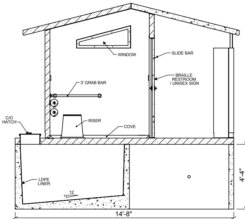
SECTION 1-1 SCALE 1 : 48
