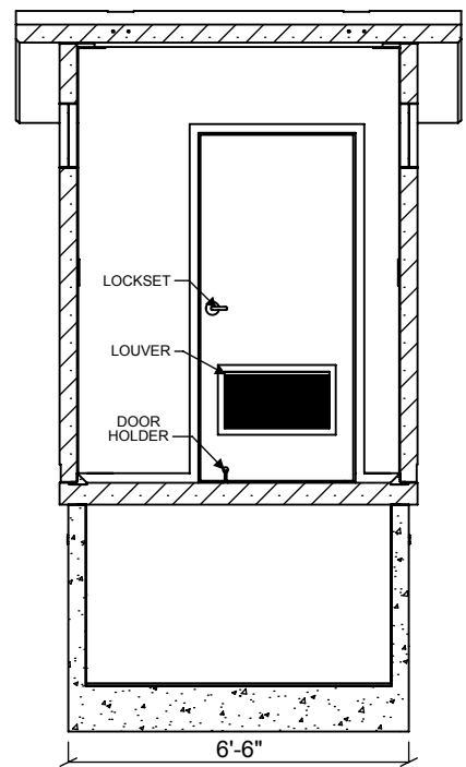
SECTION 2-2 SCALE 1 : 48
